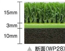
▲ 断面(WP28)
