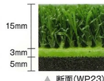
▲ 断面(WP23)
